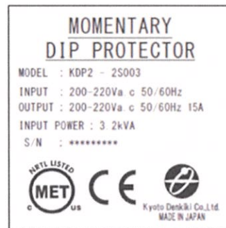
規格更新機種の製品ラベル (KDP2-2S003 の場合)
